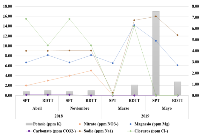
Fig. 3. Variación de los Parámetros químicos Potasio, Nitrato, Magnesio, Carbonato, Sodio y Cloruros en los puntos de salida de la planta de tratamiento de agua potable (SPT) y Red de distribución – Terminal Terrestre (RDTT), en los meses de abril y noviembre del año 2018 y los meses de marzo y mayo del 2019.
