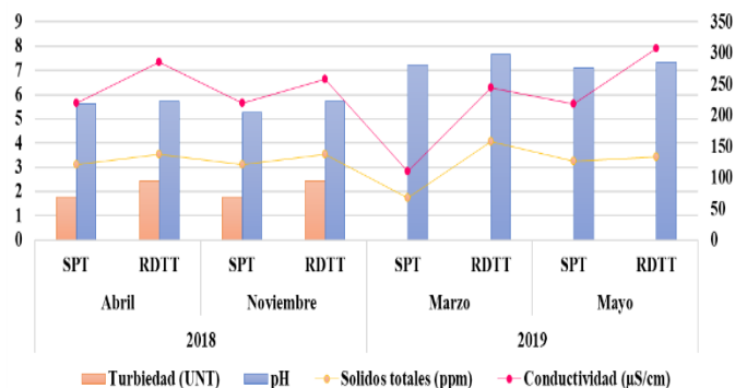
Fig. 1. Variación de los Parámetros físicos Turbiedad, pH, Conductividad y Sólidos totales en los puntos de salida de la planta de tratamiento de agua potable (SPT) y Red de distribución – Terminal Terrestre (RDIT), en los meses de abril y noviembre del año 2018 y los meses de marzo y mayo del 2019.
