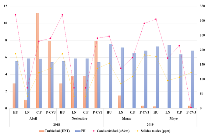
Fig. 2. Variación de los Parámetros físicos Turbiedad, pH, Conductividad y Sólidos totales en los puntos de Huayatán (HU), Laguna Negra (LN), Las Cortaderas y los Peñones (C.P), Panizaras – Canal Vicente Jiménez (P-CVJ), en los meses de abril y noviembre del año 2018 y los meses de marzo y mayo del 2019.
