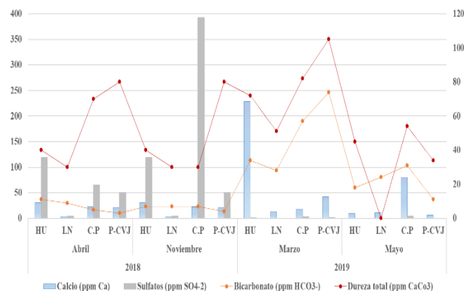
Fig. 6. Variación de los Parámetros químicos Calcio, Sulfatos, Bicarbonato, Dureza total, en los puntos de Huayatán (HU), Laguna Negra (LN), Las Cortaderas y los Peñones (C.P), Panizaras – Canal Vicente Jiménez (P-CVJ), en los meses de abril y noviembre del año 2018 y los meses de marzo y mayo del 2019.
