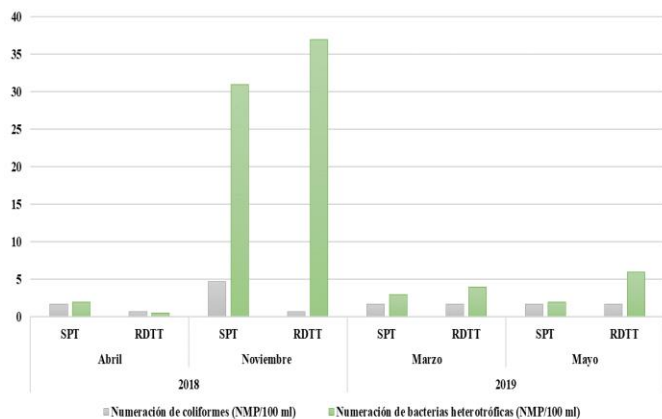
Fig. 7. Variación de los Parámetros Biológicos Numeración de coliformes y Numeración de bacterias heterotróficas en los puntos de salida de la planta de tratamiento de agua potable (SPT) y Red de distribución – Terminal Terrestre (RDTT), en los meses de abril y noviembre del año 2018 y los meses de marzo y mayo del 2019.
