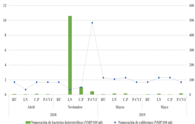
Fig. 8. Variación de los Parámetros Biológicos de Numeración de coliformes y Numeración de bacterias heterotróficas en los puntos de Huayatán (HU), Laguna Negra (LN), Las Cortaderas y los Peñones (C.P), Panizaras – Canal Vicente Jiménez (P-CVJ), en los meses de abril y noviembre del año 2018 y los meses de marzo y mayo del 2019.
