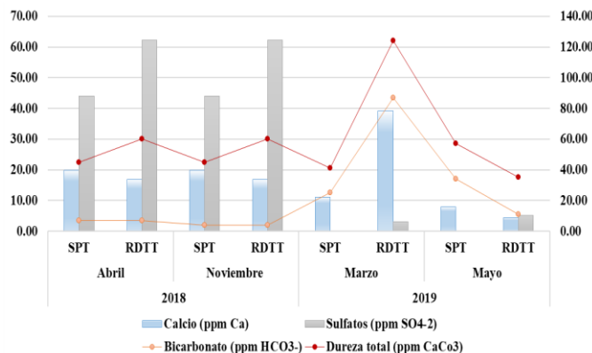
Fig. 5. Variación de los Parámetros químicos Calcio, Sulfatos, Bicarbonato, Dureza total en los puntos de salida de la planta de tratamiento de agua potable (SPT) y Red de distribución – Terminal Terrestre (RDTT), en los meses de abril y noviembre del año 2018 y los meses de marzo y mayo del 2019.
