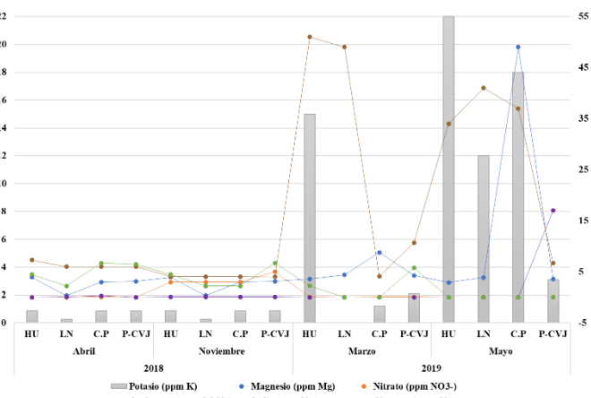
Fig. 4. Variación de los Parámetros químicos Potasio, Nitrato, Magnesio, Carbonato, Sodio y Cloruros en los puntos de Huayatán (HU), Laguna Negra (LN), Las Cortaderas y los Peñones (C.P), Panizaras – Canal Vicente Jiménez (P-CVJ), en los meses de abril y noviembre del año 2018 y los meses de marzo y mayo del 2019.
