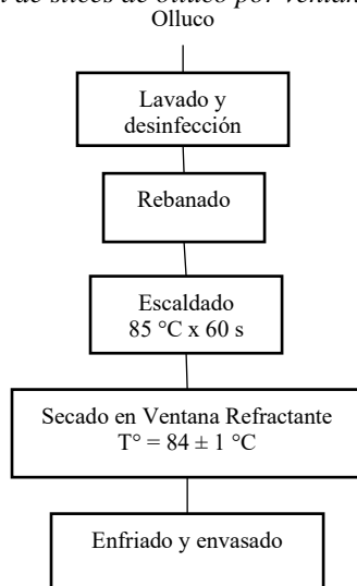
Fig. 1 Diagrama de flujo de slice de olluco
