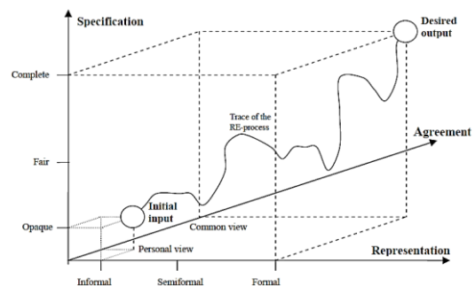
Fig. 1. NATURE framework
