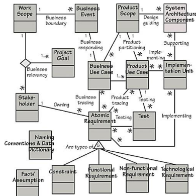
Fig. 16. Volere model
