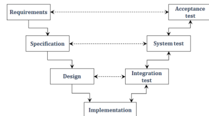
Fig. 12. Model V
